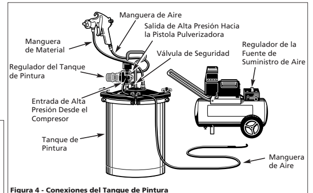
Figura 4 - Conexiones del Tanque de Pintura
