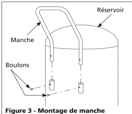
Figure 3 - Montage de manche
