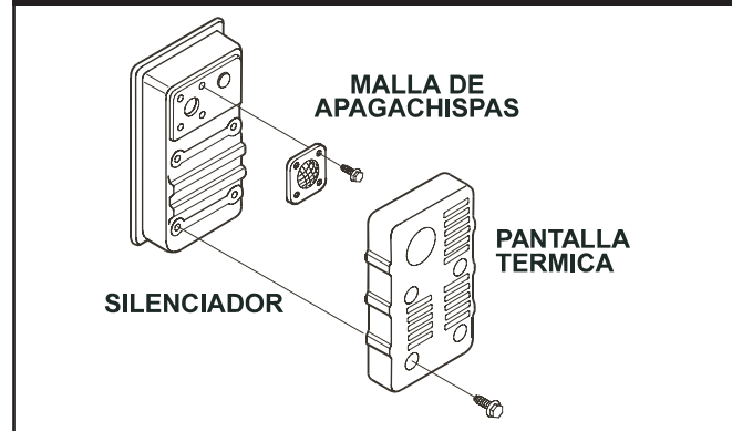
Figura 38 — Servicio al Pantalla Apagachispas
