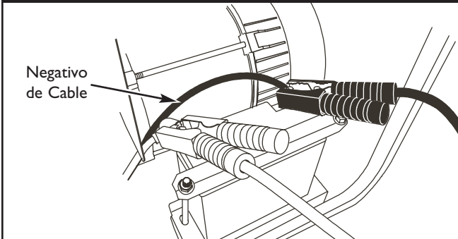
Figura 25 — Conexiones del Cable de Puente
