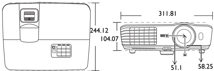
MX717
