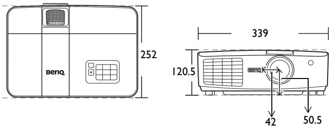
MX717
