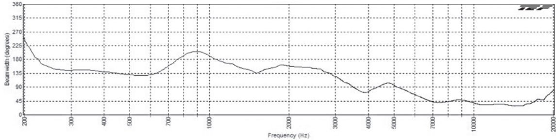
FC104 Beamwidth (-6dB)
