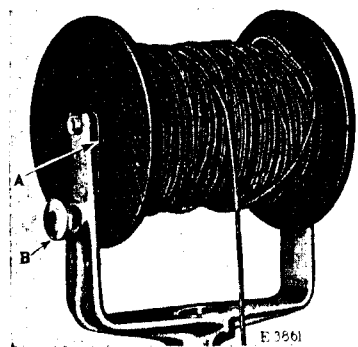
FIG. 30. BRAID SPOOL TENSION
