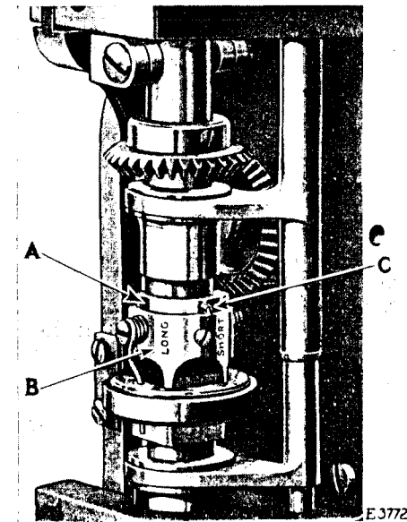
FIG. 29. STITCH REGULATOR
