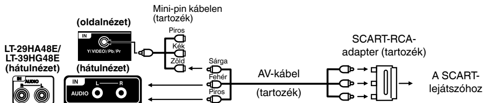
Csatlakozás SCART-lejátszóhoz
